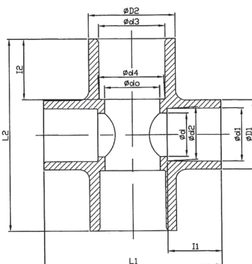
異徑十字通
