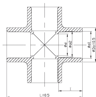
十字通
